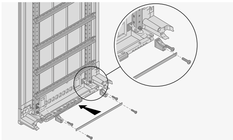
Exemple de montage horizontal
