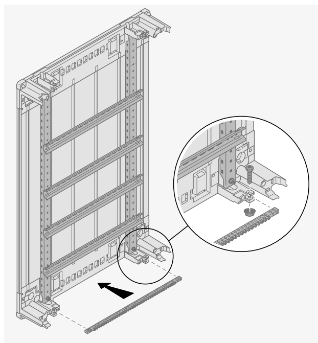
Exemple de montage vertical
