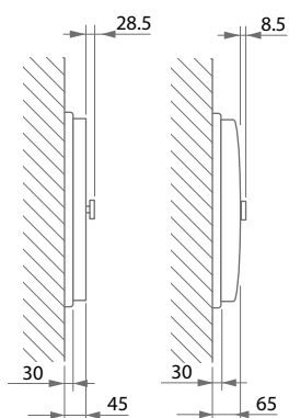
Porte plate Porte galbée
