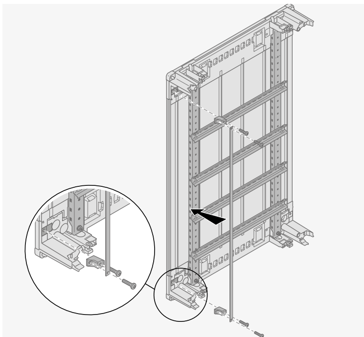
Exemple de montage vertical
